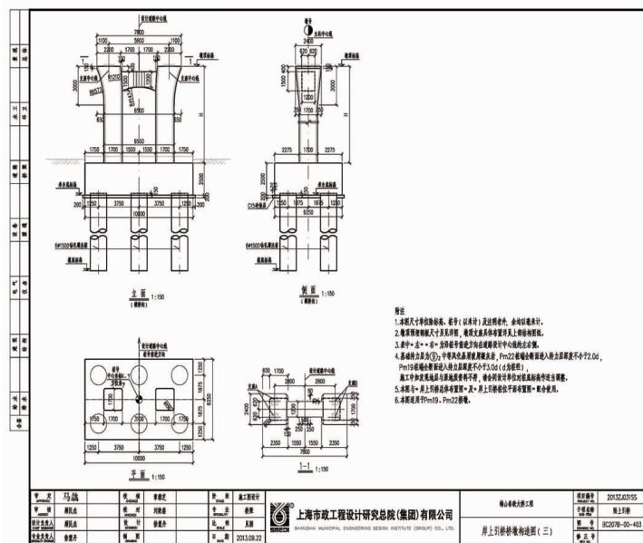
图12 二维出图
