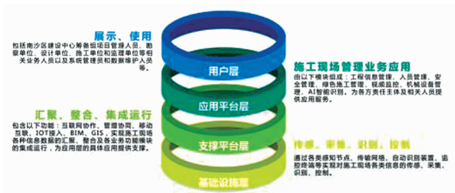
图2 智慧工地系统架构
