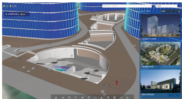
图 13 Catia 幕墙模型和 Revit 土建模型的合模
