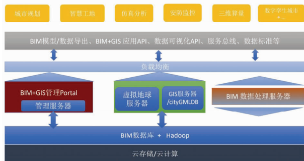
图 12 BIM + 3D GIS 的大数据平台架构
