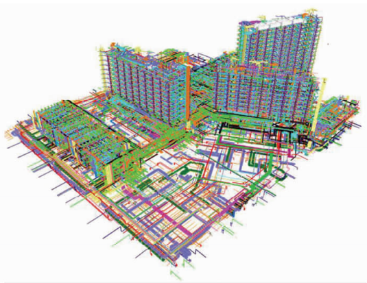
图 7 机电专业整合模型
