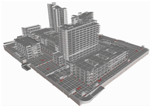
图 5 土建专业整合模型
