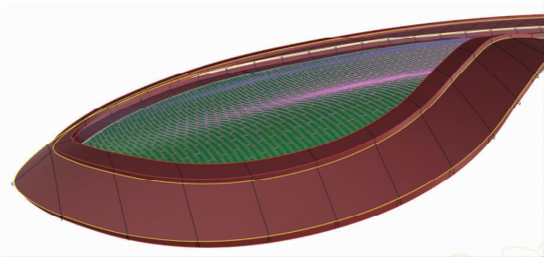
图4 檐口造型与吊顶曲面关系
