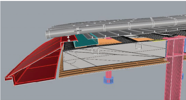
图2 檐口处剖面
