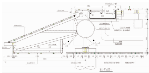
图6 檐口造型图
