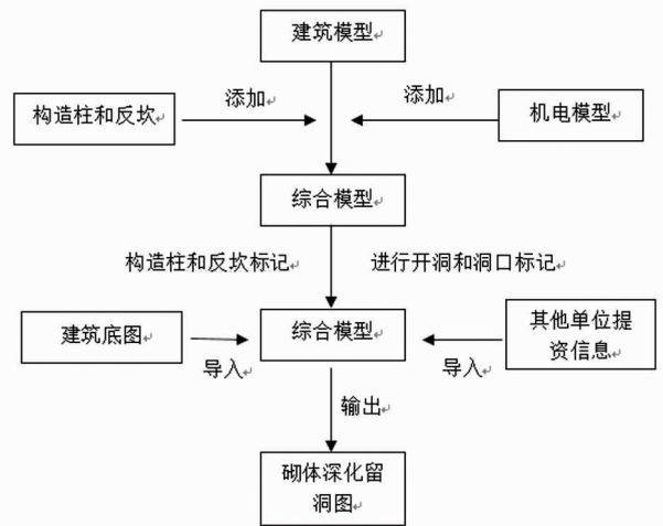
图 3 流程图
